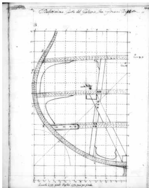
fig. 5 - ROBERT DUDLEY, Il Perfettissimo Garbo del Galeone San Giovanni Battista , Londra, British Museum, add. ms. 22811
