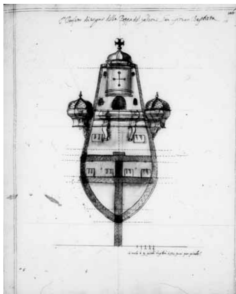
fig. 4 - ROBERT DUDLEY, Il Perfetto disegno della Poppa del Galeone San Giovanni Battista , Londra, British Museum, add. ms. 22811
