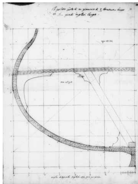
fig. 8 - ROBERT DUDLEY, Il perfetto Garbo di un pinnaccio... , Londra, British Museum, add. ms. 22811
