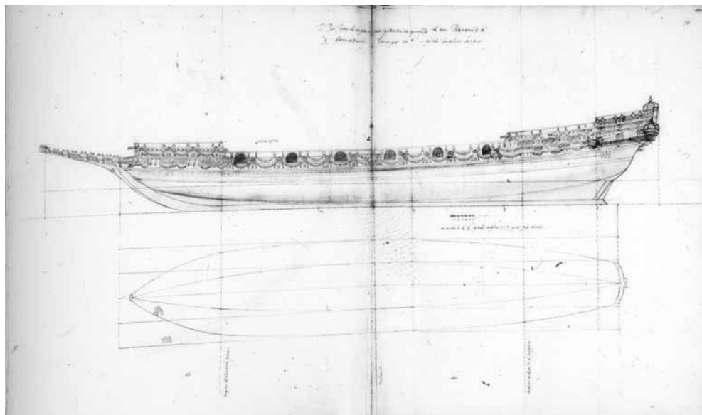
fig. 6 - ROBERT DUDLEY, Il Perfetto disegno con pianta e profilo di un Pianaccio... , Londra, British Museum, add. ms. 22811
